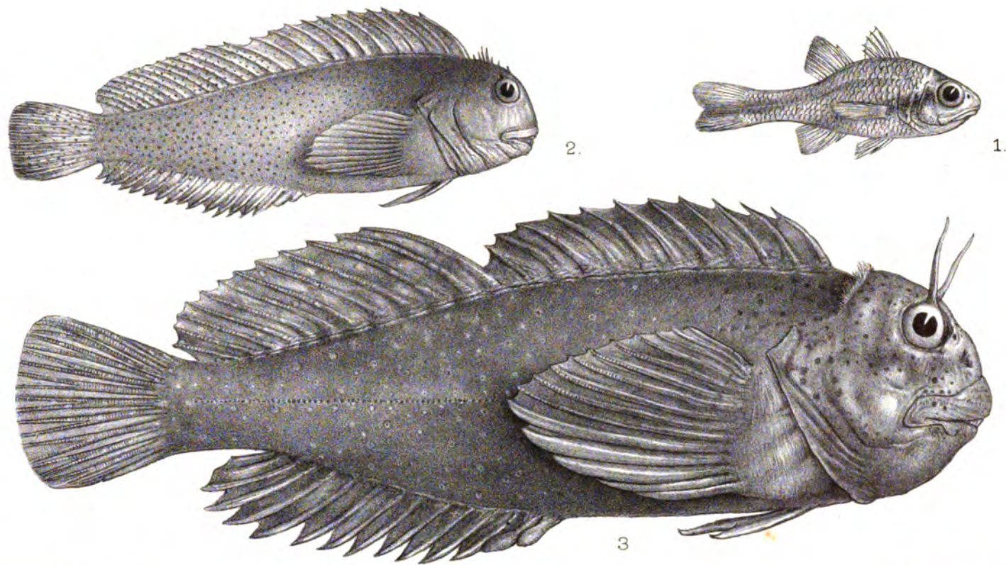
1. APOGON WARRENI. 2. BLENNIUS PUNCTIFER. 3. SALARIAS KOSIENSIS.
